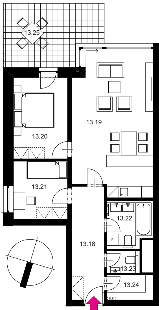
půdorys bytové jednotky 3+kk v 1.NP
